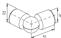
Connettore ad angolo regolabile per profilo Ø16 Adjustable angle connector for profile Ø16
