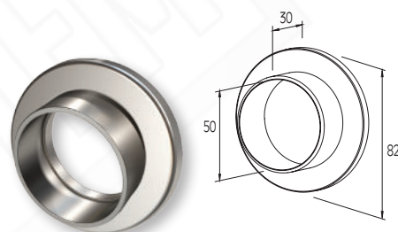
Fissaggio a parete per corrimano Ø50 con cover Wall cover for handrail Ø50 with cap
