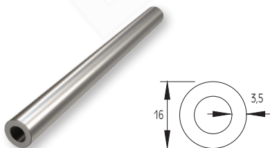
Profilo Ø16x3.5 Profile Ø16X3.5
