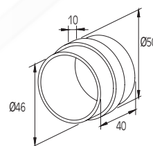
Connettore per corrimano Ø50 (interno) Connector for handrail Ø50 (internal)
