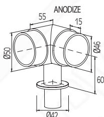
Connettore 90° per corrimano Ø50 Connector 90° for handrail Ø50
