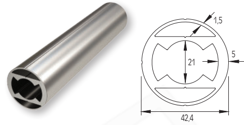
Colonna rinforzata Ø42 Reinforced column Ø42
