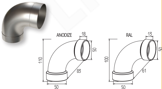
Connettore 90° per corrimano Ø50 Connector 90° for handrail Ø50
