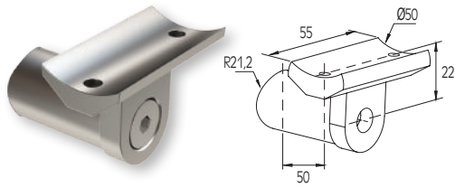
Supporto esterno per corrimano Ø50-colonna Ø42 External support for handrail Ø50-column Ø42
