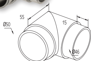
Connettore 90° per corrimano Ø50 Connector 90° for handrail Ø50
