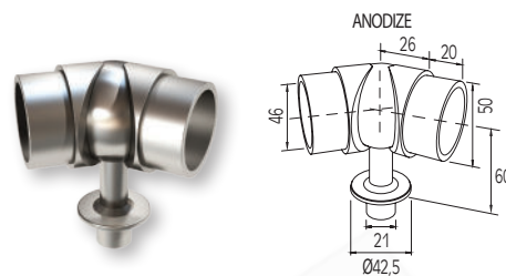
Connettore ad angolo regolabile per corrimano Ø50 - colonna Ø42 Adjustable corner railtop connector
