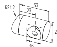
Connettore per F50-100 con profilo Ø16 Connector for F50-100 column with guide Ø16
