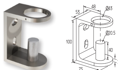
Supporto per fissaggio frontale per colonne F50-100/103 External support for F50-100/103 columns
