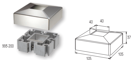
Piede per colonna 40x40 Support foot for 40x40 column Codice / Code 4122
