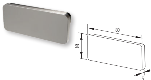
Coperchio per corrimano F50-201 End cap for F50-201 handrail
