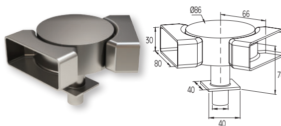
Connettore ad angolo regolabile per corrimano 80x30 con colonna F50-102 Adjustable corner connector for 80x30 handrail with F50-102 column
