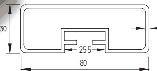
Corrimano 30x80 Handrail 30x80
