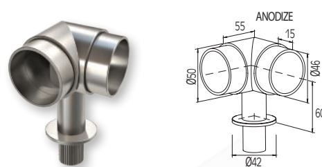
Raccordo angolo 90° per corrimano Ø50 con colonna F50-100 Connector 90° for handrail Ø50
