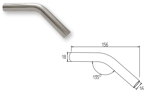
Connettore 135° per profilo Ø16 Connector 135° for profile Ø16
