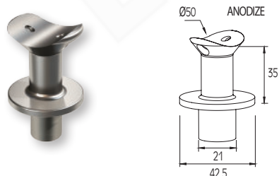
Connettore per corrimano Ø50 con colonna Ø42 Connector for handrail Ø50 with column Ø42
