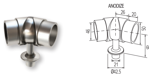
Connettore ad angolo regolabile per corrimano Ø50 con colonna Ø42 Adjustable corner Ø50 railtop connector
