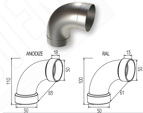
Connettore 90° per corrimano Ø50 Connector 90° for handrail Ø50
