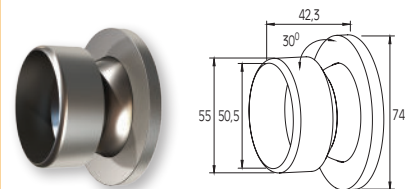
Cover a parete orientabile per corrimano Ø50 Wall cover for handrail Ø50 Codice / Code 4518
