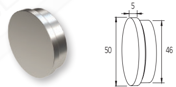
Coperchio per corrimano F50-200 (piatto) End cap for F50-200 handrail (flat) Codice / Code 4453
