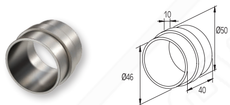
Connettore per corrimano Ø50 (interno) Connector for handrail Ø50 (internal)
