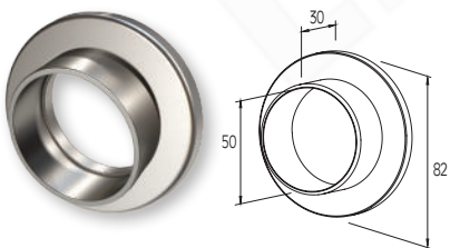
Fissaggio a parete per corrimano Ø50 Wall cover for handrail Ø50 Codice / Code 4509Z
