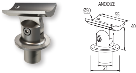
Connettore per corrimano Ø50 con colonna Ø42 (scale) Connector for handrail Ø50 with column Ø42 (stairs) Codice / Code 4316
