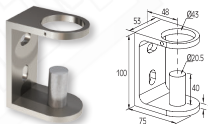
Supporto per fissaggio frontale per colonne F50-100 e F50-103 External support for F50-100/103 columns
