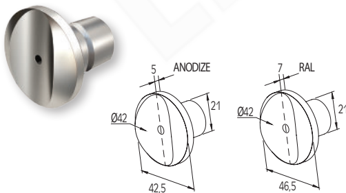
Connettore per colonna F50-100 con colonna F50-100 Connector for column with column F50-100
