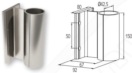
Supporto per fissaggio frontale per colonna Ø42 External support for column Ø42
