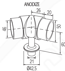
Connettore ad angolo regolabile per corrimano Ø50 con colonna Ø42 Adjustable corner connector for column Ø42
