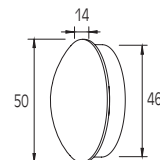
Coperchio per Corrimano F50-200 End cap for F50-200 handrail
