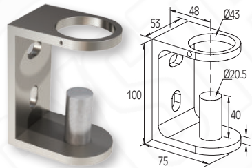
Supporto per fissaggio frontale per colonne F50-100 / 103 External support for F50-100/103 columns
