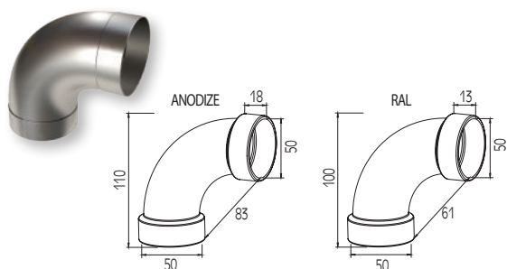
Connettore 90° per corrimano Ø50 Connector 90° for handrail Ø50
