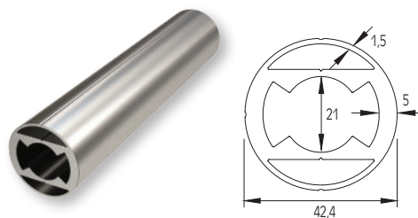
Colonna rinforzata Ø42 Reinforced column Ø42
