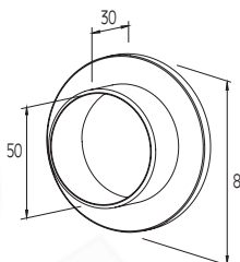
Fissaggio a parete per corrimano Ø50 Wall cover for handrail Ø50 with cap
