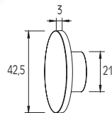
Coperchio per colonna F50-100 End cap for F50-100 column
