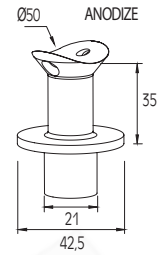
Connettore per corrimano Ø50 con colonna Ø42 Connector for handrail Ø50 with column Ø42
