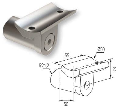
Supporto esterno per corrimano Ø50-colonna Ø42 External support for handrail Ø50-column Ø42
