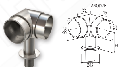
Raccordo angolo 90° per corrimano Ø50 con colonna F50-100 Connector 90° for handrail Ø50
